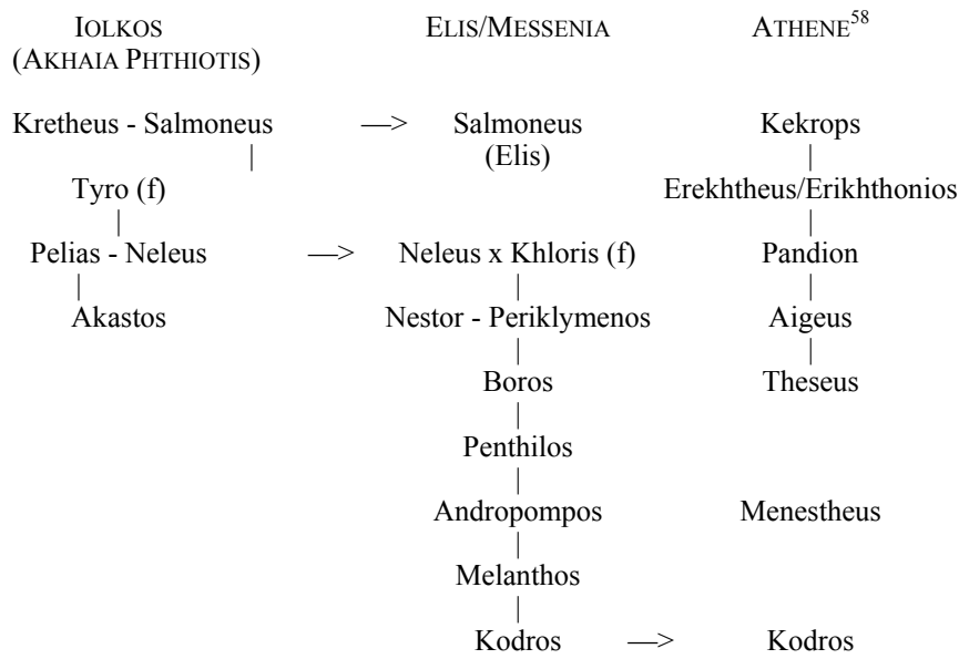
Fig. 2. Stemmata (continued).
